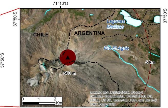
Sernageomin - Red Nacional de Vigilancia Volcánica Mapa de Peligros Volcánicos - Mayo 2021 Volcán Copahue - Alerta Verde
